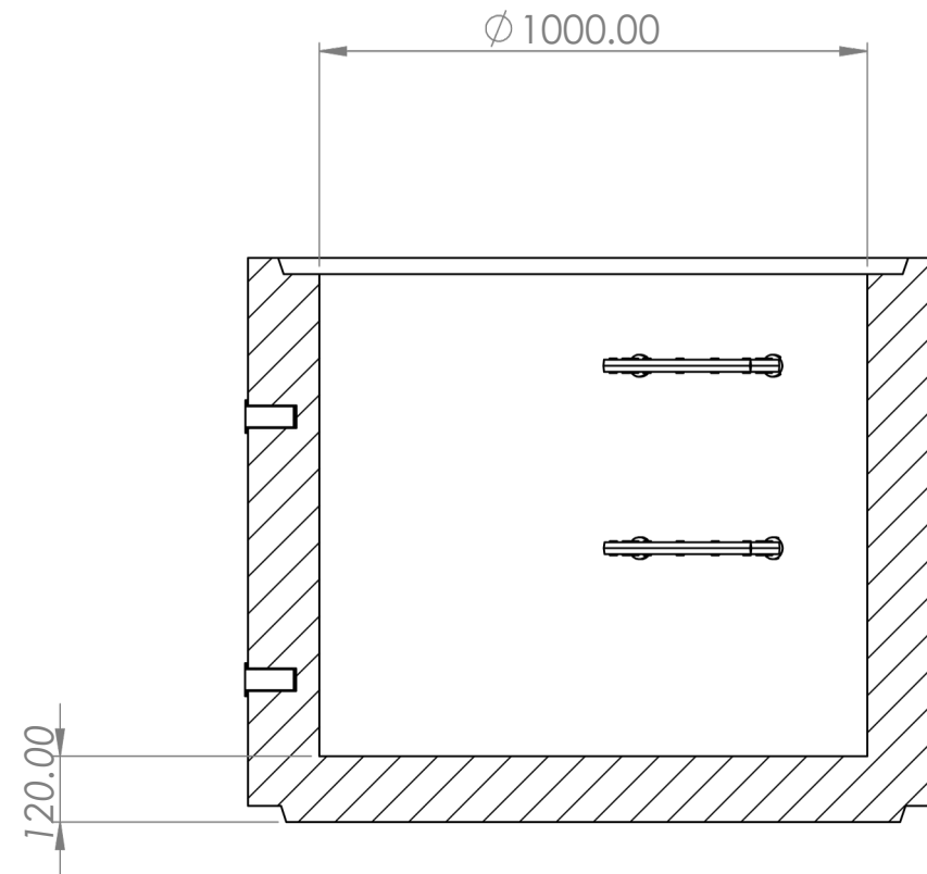
SECTION A-A SCALE 1 : 15
