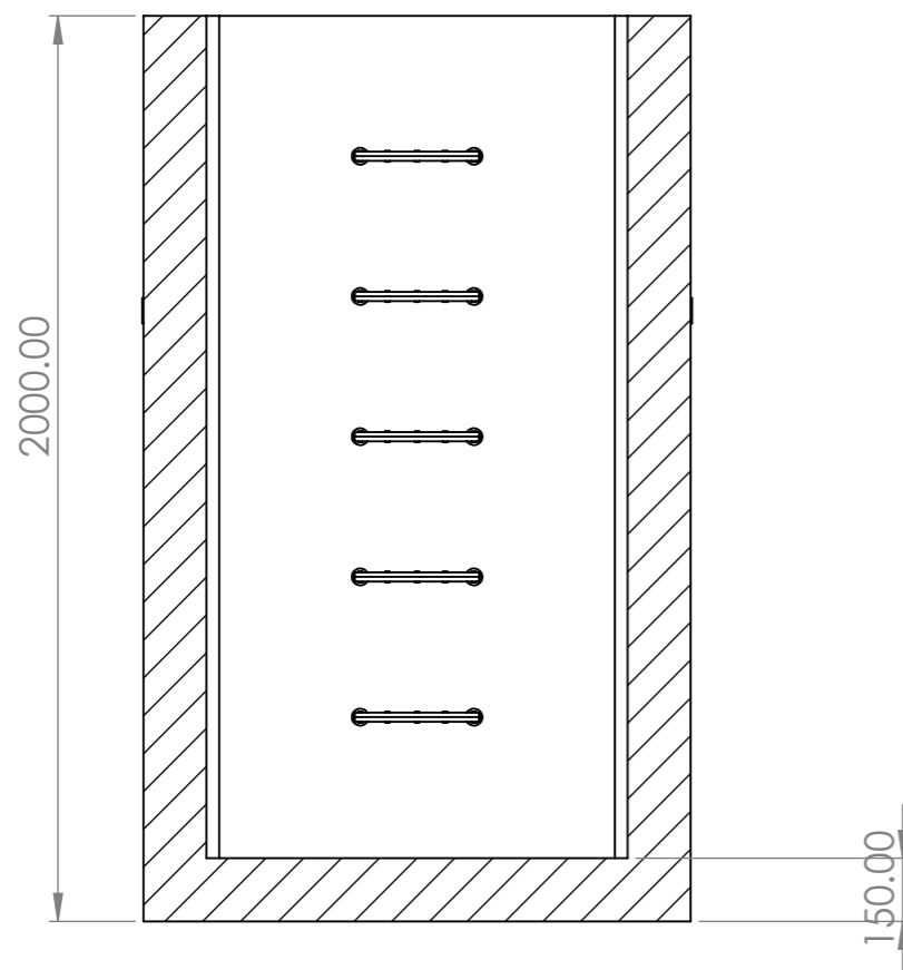
SECTION A-A SCALE 1 : 20
